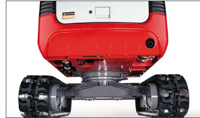
Große Bodenfreiheit, geschlossener und daher besonders geschützter Unterwagen.
